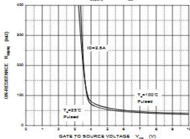
R_{DS(on)} — V_{GS}
