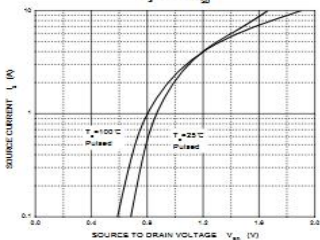
I_S — V_{SD}
